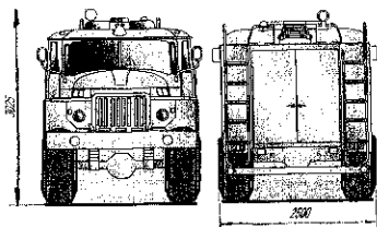
Рис.4 АЦ-4,0-40(Упан-5557)-9Б
