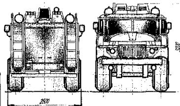
Рис.5 АЦ-5,0-40(Упан-5557)-11Б
