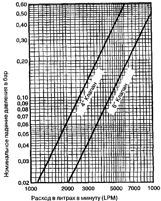
Зависимость падения номинального давления от скорости потока.
