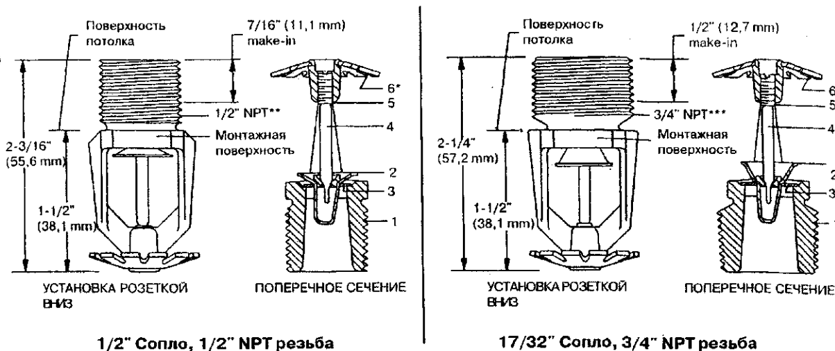
Рис. А Универсальные спринклеры модели А
