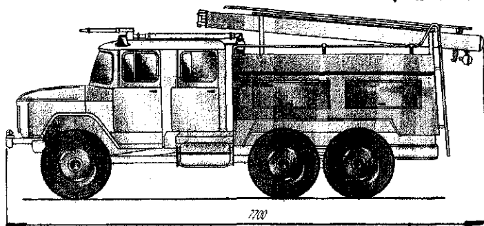
Рис.1 АЦ-2,5-40(ЗИП-131)-БВР
