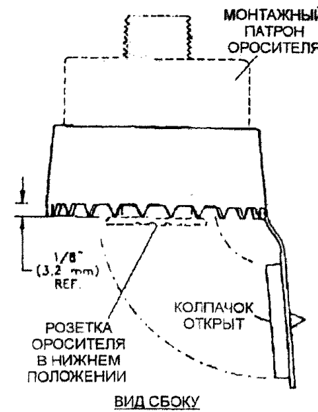
Рис.4 Защитный колпак
