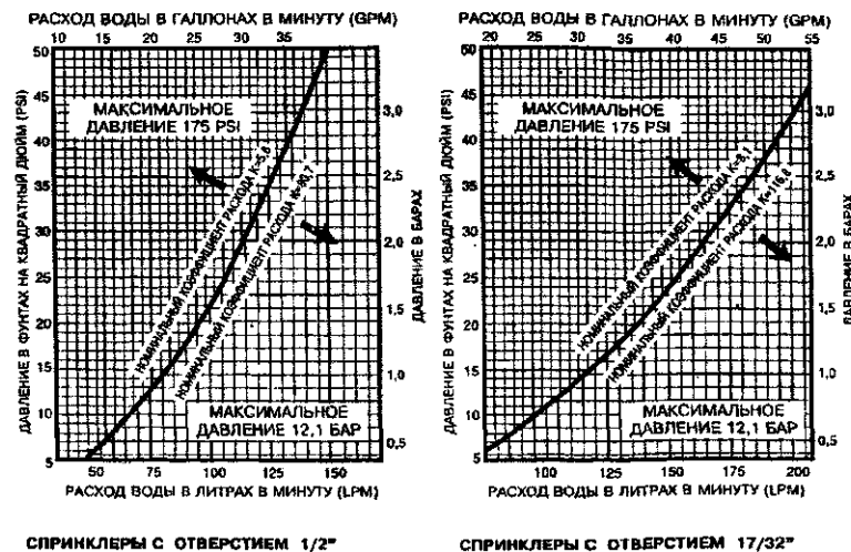
Рис. В. Кривая номинального расхода
