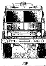
Рис.6 АЦ-5,0-40(КамАЗ-43114)-20БР
