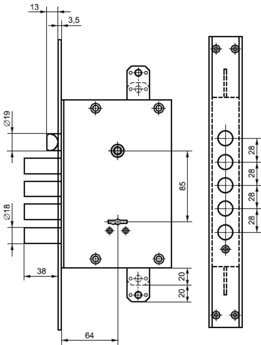
Рисунок Б.6 - Пример сувальдного врезного замка типа 3B11
