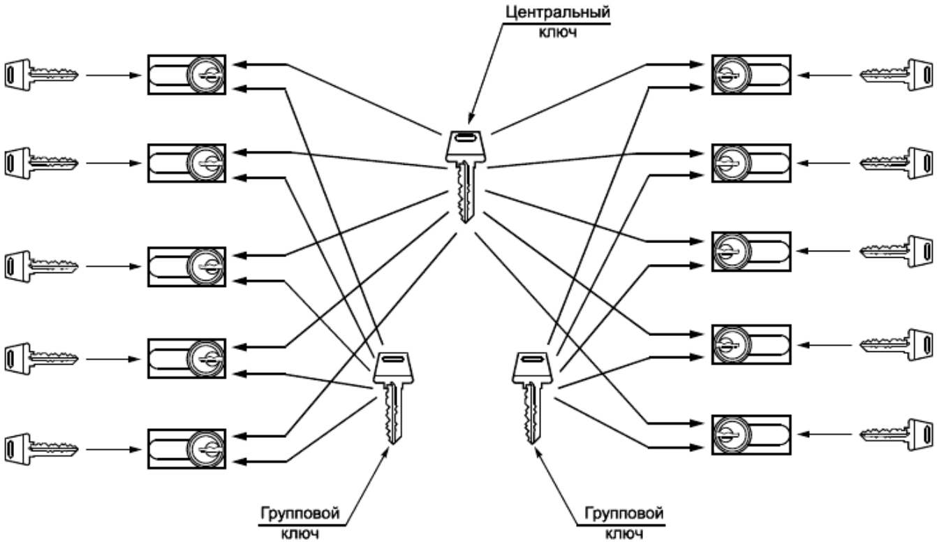
Рисунок А.4 - Система цилиндрических механизмов с центральным ключом - набор, состоящий не менее чем из двух систем цилиндрических механизмов с групповым ключом,
