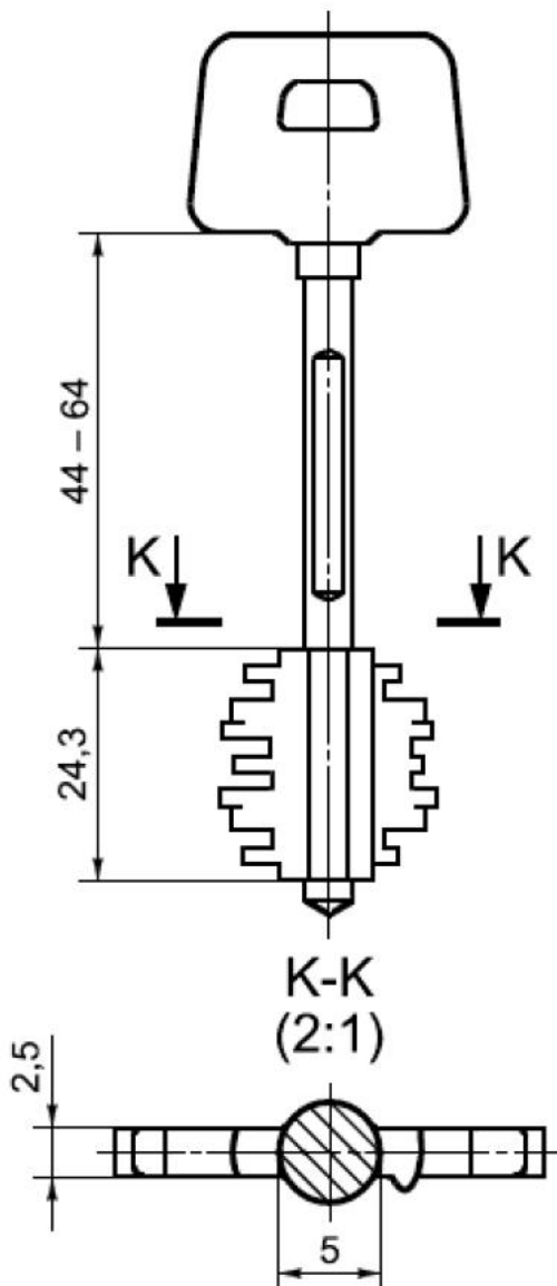
Рисунок Б.20 - Пример ключа сувальдного замка
