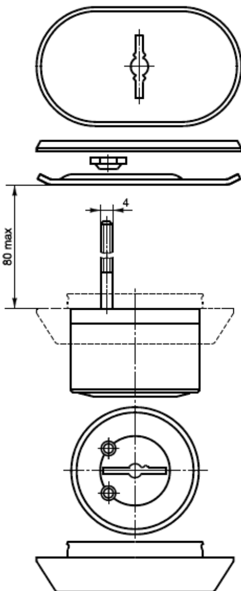
Рисунок Б.18 - Пример запорной планки для накладного замка
