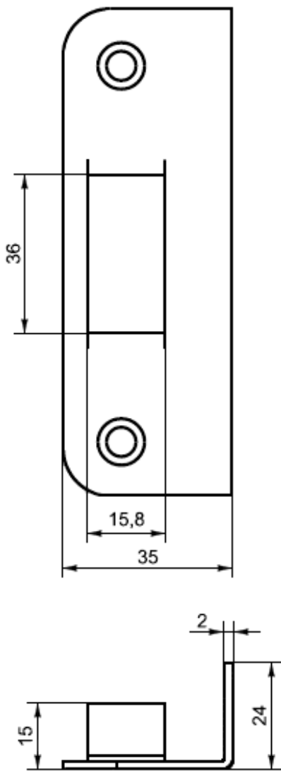
Рисунок Б.16 - Пример запорной угловой планки
