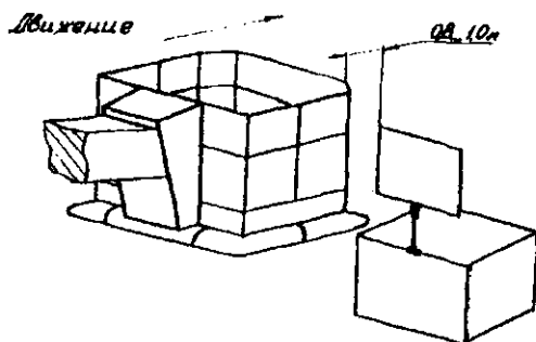
Рисунок 1. Схема положения люльки АКК относительно приспособления "щит-препятствие" при перемещении колен стрелы относительно друг друга
