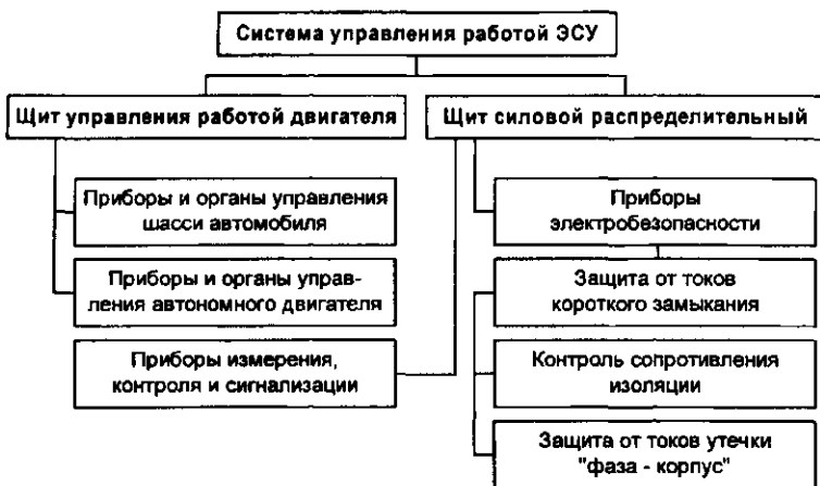
Рисунок 1. Структура системы управления работой ЭСУ автомобилей связи и освещения
