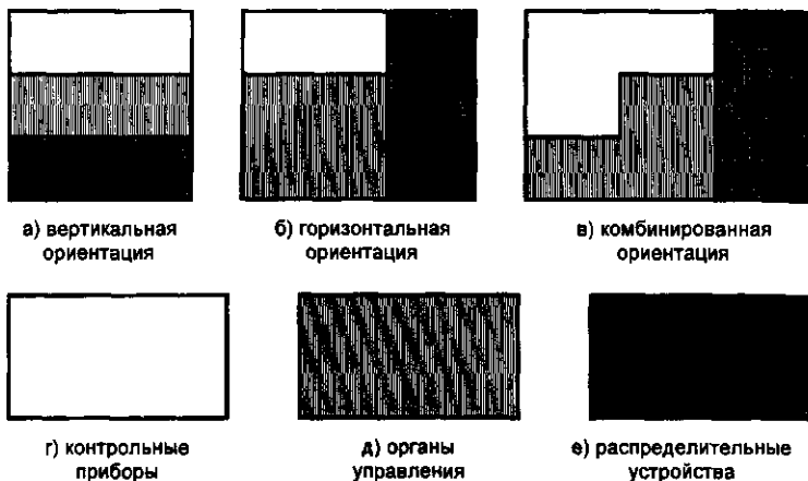
Рисунок 2. Варианты компоновки щитов управления
