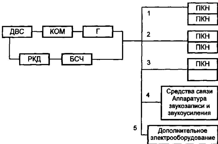
Рисунок 3 Схема развертывания стационарных и переносных приемников электроэнергии АСО
