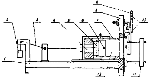
Рис. 1. Принципиальная схема установки для определения устойчивости материалов и тканей СИЗР к воздействию теплового потока:
