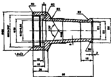
Рис. 2.1. Ствол-водомер: 1 - насадок мерный; 2 - ствол в сборе; 3 - штуцер для манометра
