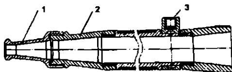
Рис. 2.1. Ствол-водомер: 1 - насадок мерный; 2 - ствол в сборе; 3 - штуцер для манометра
