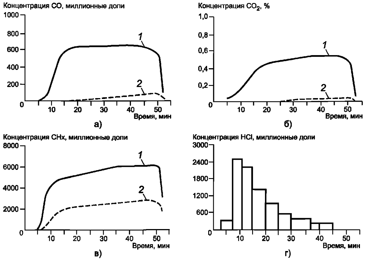
Рисунок 14 — Концентрации газов: а — CO, б — CO 2 , в — CH x , г — HCl, в вентиляционном пространстве 1 и комнате 2 при полномасштабных огневых испытаниях с использованием в качестве топлива только проводов с ПВХ-изоляцией, расположенных в вентиляционном пространстве [19]
