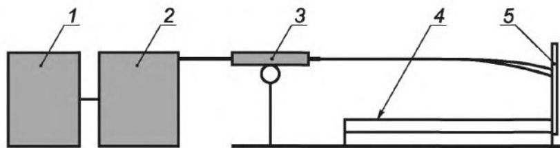
1 — емкость с пенообразователем; 2 — насосная установка; 3 — пенный ствол; 4 — противень с горючей жидкостью; 5 — экран для сбора пены
