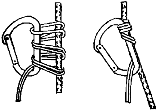
Рисунок 10 — Узел Бахмана
