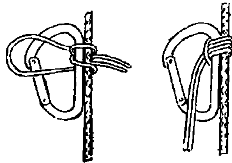
Рисунок 11 — Карабинный узел
