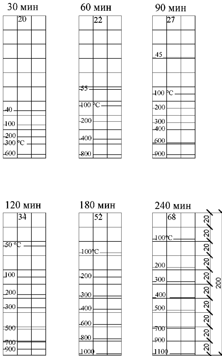
Рисунок И.12 - Плита из тяжелого бетона толщиной 200 мм при нагреве с одной стороны
