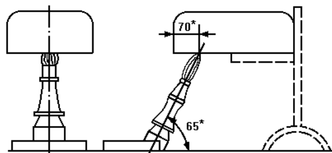
Рис. 2. Расположение горелки при горизонтальном расположении образца
