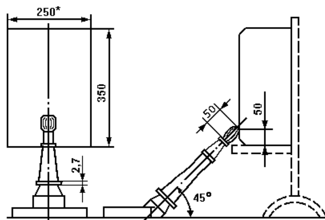
Рис. 1. Расположение горелки при вертикальном расположении образца
